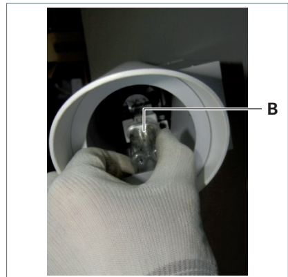
Fig. 3: Lampe einsetzen.
