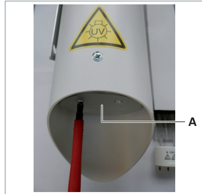
Fig. 1: Retirer le panneau de protection des tubes.
