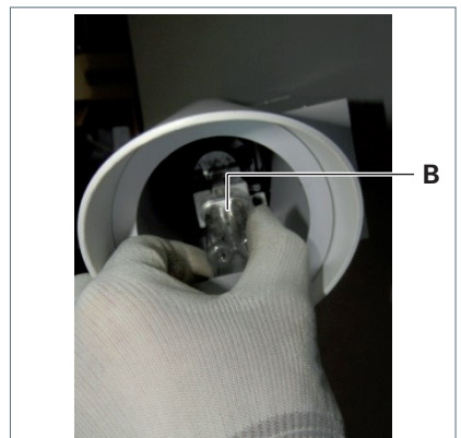
Fig. 3: Insert lamp.
