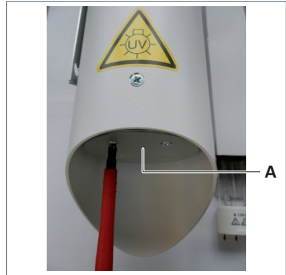
Fig. 1: Lampenabdeckung entfernen.
